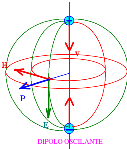
DIPOLO OSCILANTE
