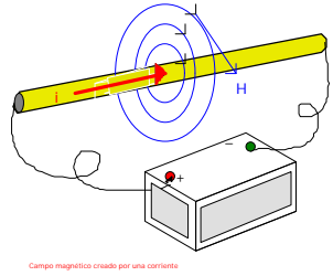
Campe magnetico creado por una corriente
